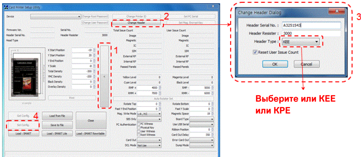
Рис. 67 Установка печатной головки
