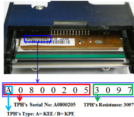
Рис. 66 Термопечатная головка
