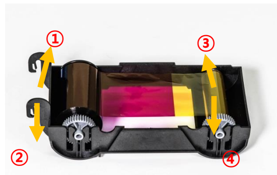
Рис. 11 Установка ленты 2
