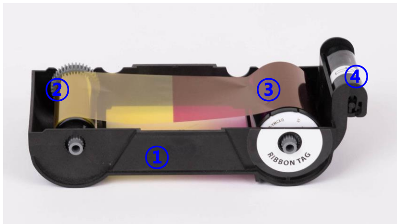
Рис 5 Характеристики съемного картриджа для лент
