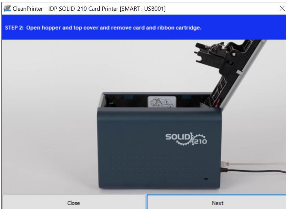
Рис. 61 Очистка принтера Шаг 2
