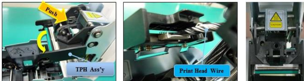
Рис. 68 Замена печатной головки
